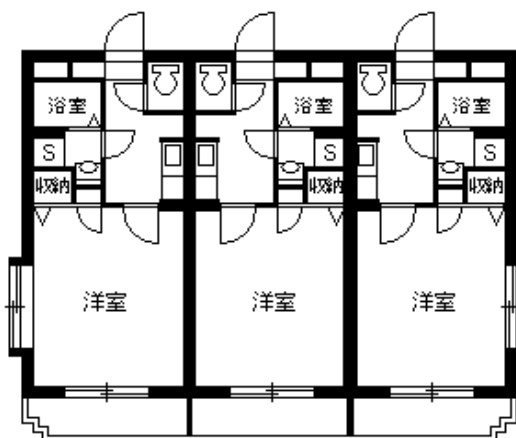
2F~5F間取図
